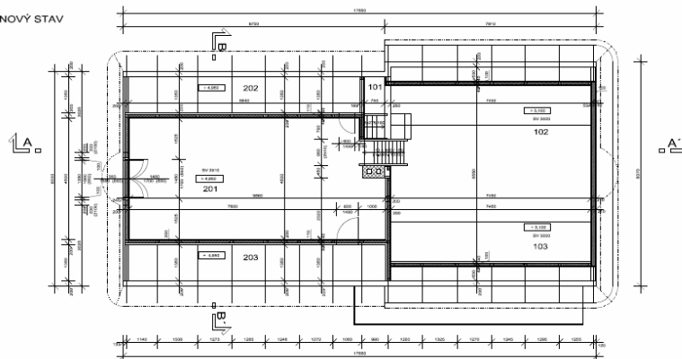
PŮDORYS 3.N.P. - NOVÝ STAV
