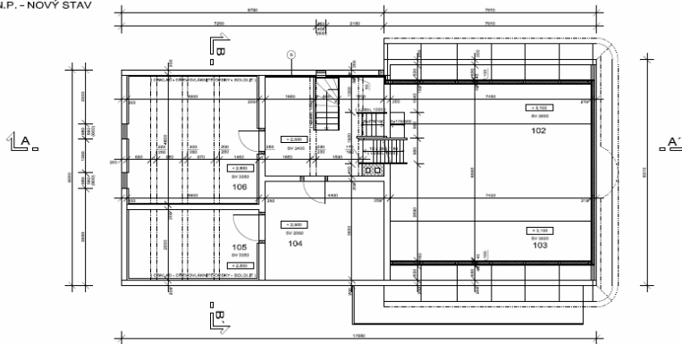
PŮDORYS 2.N.P. - NOVÝ STAV
